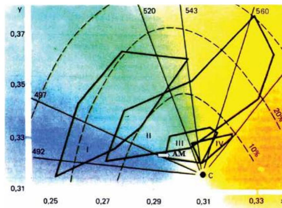
Figura 5. Gráfico colorimétrico de las amazonitas: pegmatitas de la Península de Kola (I) y de Urales (II); granitos de Transbaikal (III) y Kazajstan (IV). AM-amazonita mexicana. Modificada de Ostrooumov (1987).
